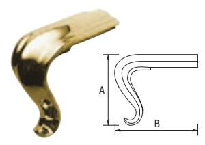
H1600LT Cap Rail Lamb Tongue End
